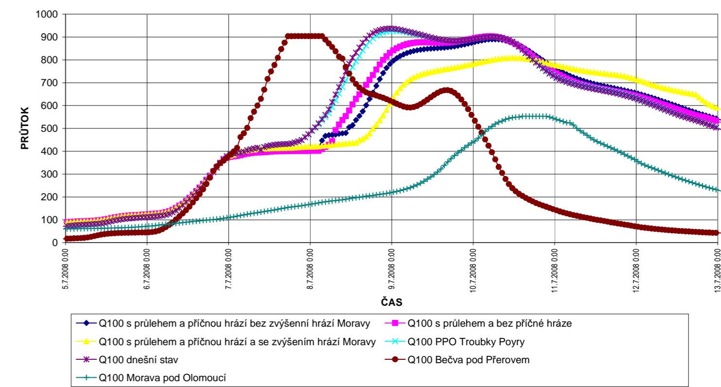
POROVNÁNÍ VLIVU VARIANT PPO PRO POVODĚNÍ Q100 NA PRŮTOK V MORAVĚ V PROFILU TRATI KOJETÍN-PREROV
