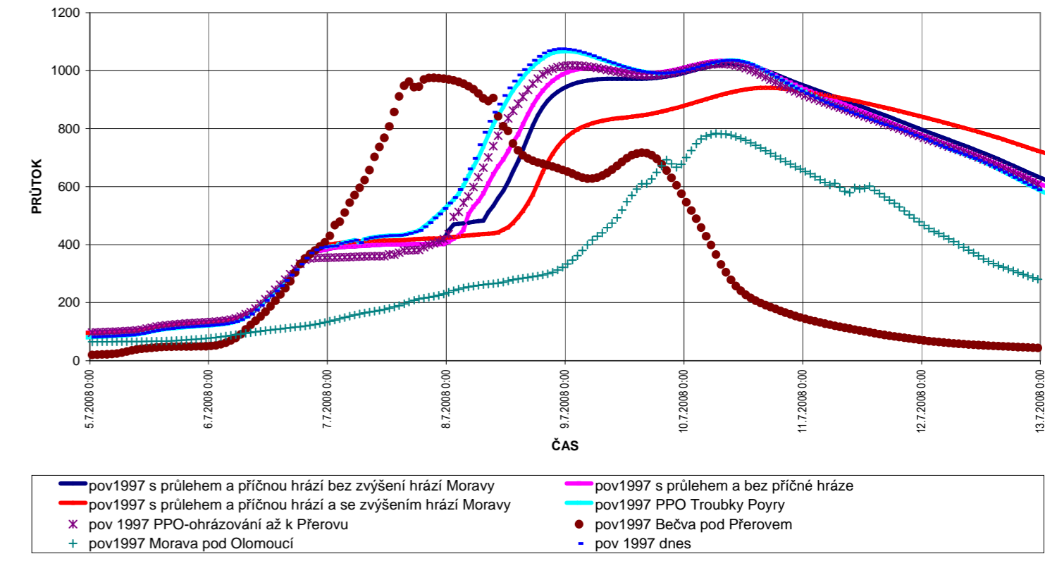
POROVNÁNÍ VLIVU VARIANT PPO PRO POVODĚNÍ 1997 NA PRŮTOK V MORAVĚ V PROFILU TRATI KOJETÍN-PREROV
