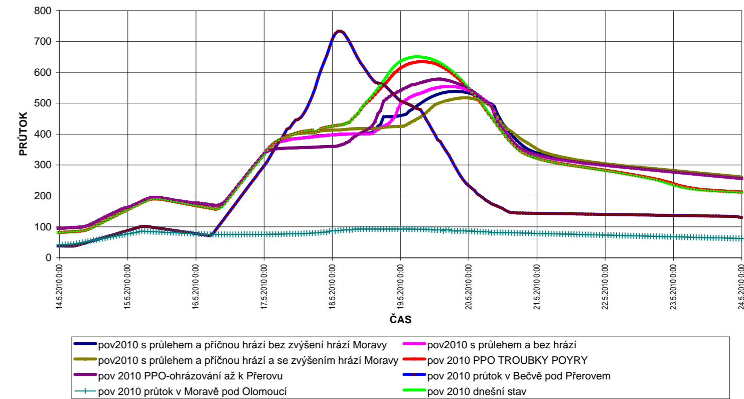
POROVNÁNÍ VLIVU VARIANT PPO PRO POVODĚNÍ 2010 NA PRŮTOK V MORAVĚ V PROFILU TRATI KOJETÍN-PREROV
